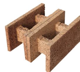
DOPPIO BLOCCO ACUSTICO 22/15
