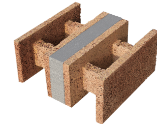
DOPPIO BLOCCO ACUSTICO 22/15 CON 8CM. DI GRAFITE
