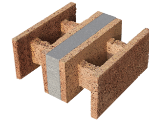
DOPPIO BLOCCO ACUSTICO 22/15 CON 8CM. DI GRAFITE
