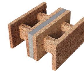
DOPPIO BLOCCO ACUSTICO 22/15 CON 4CM. DI GRAFITE
