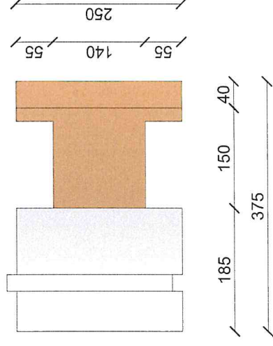
VISTA LATERALE
