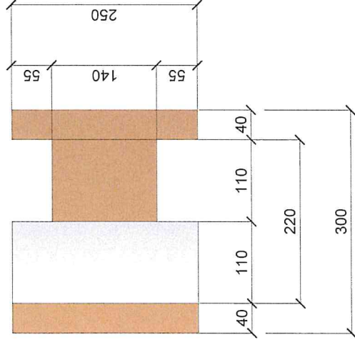
VISTA LATERALE
