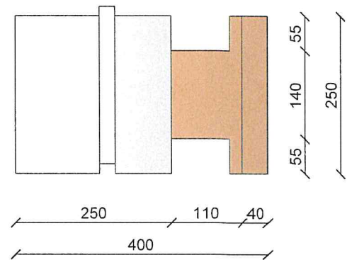
VISTA INTERNA
