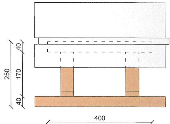
VISTA INTERNA
